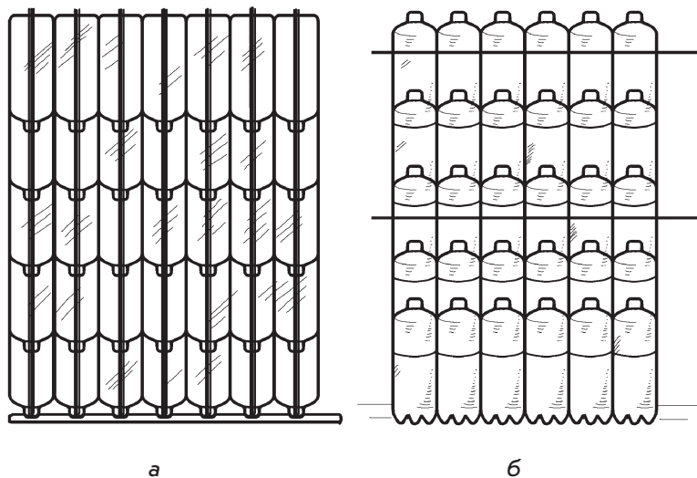
Рис. 1. Стены из пластиковых бутылок в виде: а — нанизывания; б — «бревнышек»
