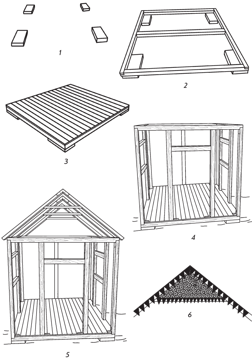
Рис. 4. Этапы строительства игрового домика (вариант 1)
