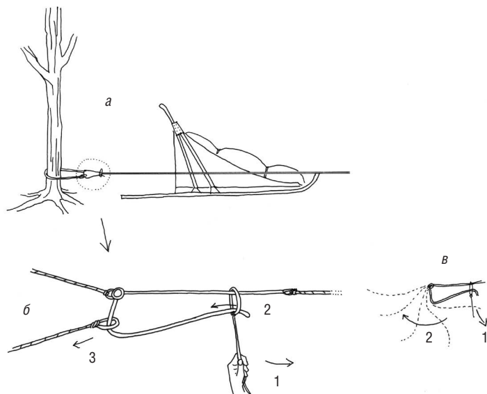
Сани удерживаются на месте с помощью веревки, снабженной фиксатором а) фиксатор; б) деталь фиксатора: 1 — нужно дернуть за веревку; 2 — фиксатор открывается; 3 — веревка отпущена; в) функционирование фиксатора
